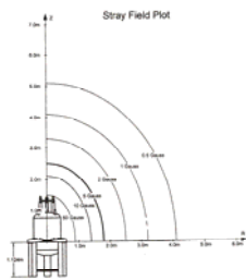
Das Erdmagnetfeld hat eine Stärke von 30-60 \mu\text{T} (0.3-0.6 Gauss)
